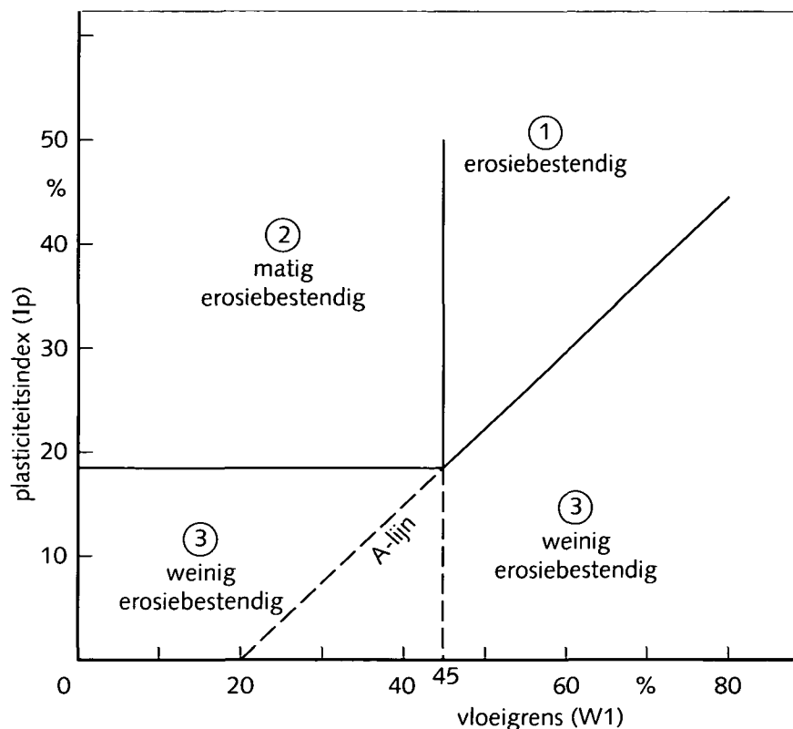
Figuur 5.1 Erosiebestendigheid uitgezet in het plasticiteitsdiagram; de vergelijking van de A-lijn is I_p = 0.73 * (w_1 - 20)
